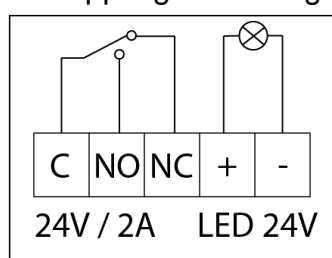
Nyckelbrytare NB-1
